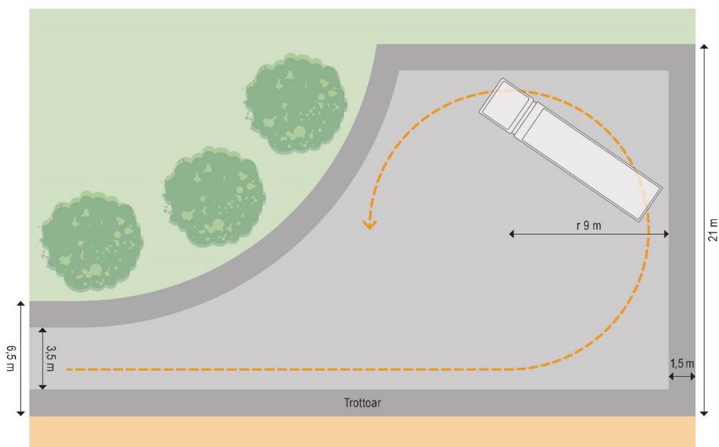
Figur 1: Dimensionering av vändplats. (Illustration: Avfall Sverige)
